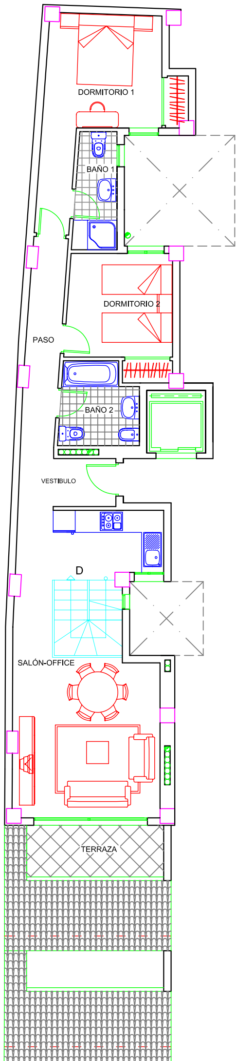
PLANTA SOBREATICO D
